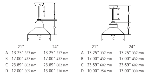
PENDANT MOUNT P(X)
